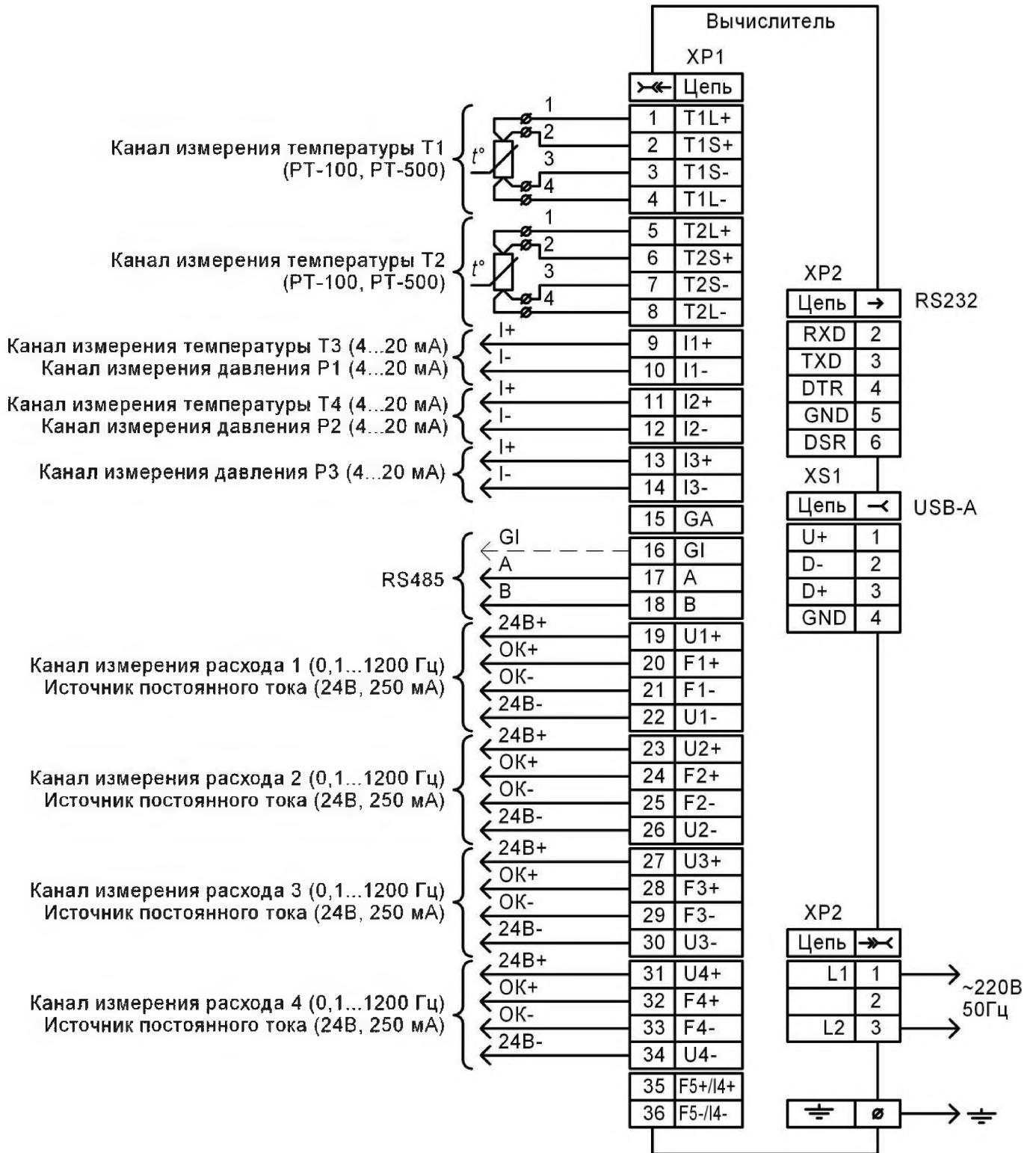
Схема подключений вычислителя
